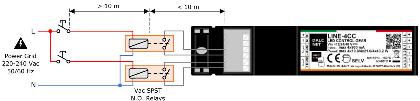
Figura 7: Collegamento del Comando Locale per lunghe distanze
