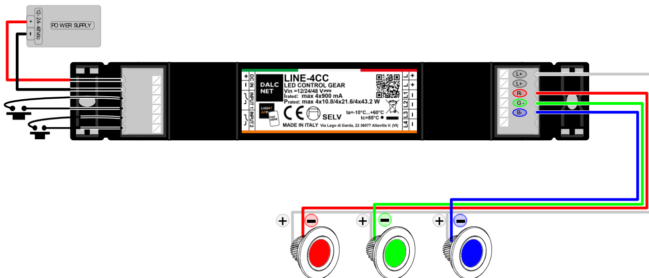
Figura 4: Schema di collegamento per carico RGB
