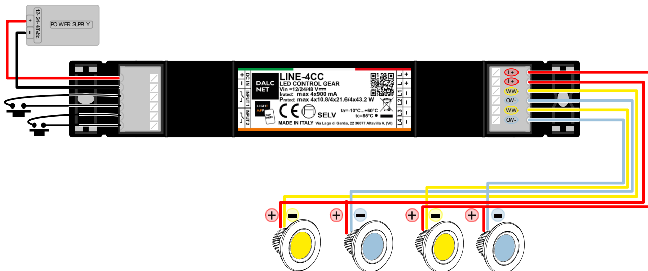
Figura 3: Schema di collegamento per carichi LED Tunable-White
