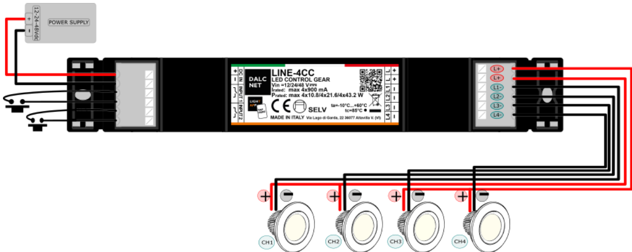
Figura 2: Schema di collegamento per carichi LED Bianchi o Monocolore
